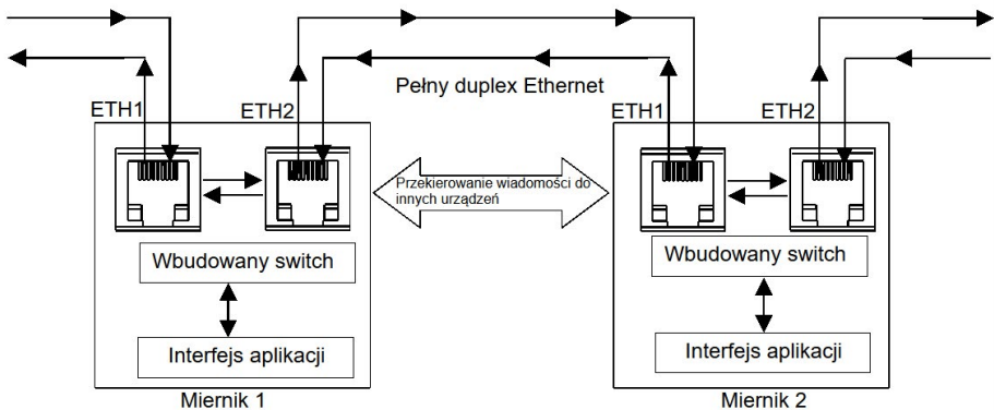
Rys. 45. Konfiguracja sieci Ethernet z 2-portowym switchem Ethernet
