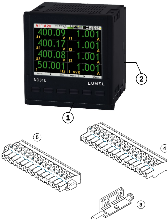
Rys. 1. Zestaw miernika
