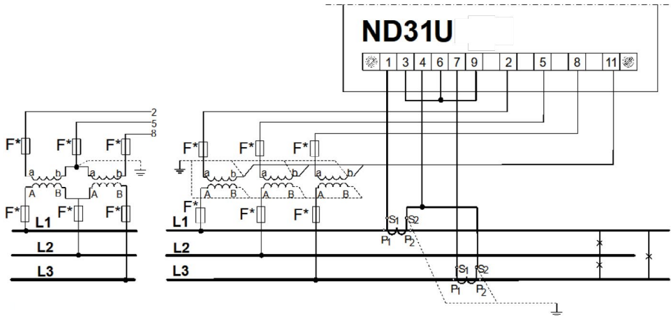
Rys. 7. Podłączenia sygnałów wejściowych w sieci trójfazowej 3 – przewodowej
