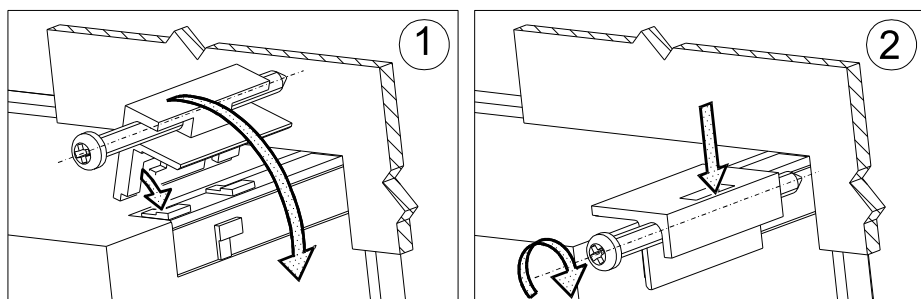
Rys. 2. Mocowanie miernika
