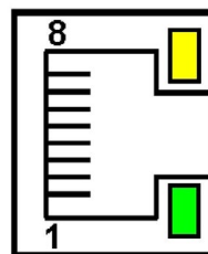
Rys. 46. Widok i numeracja pinów gniazda RJ45 miernika
