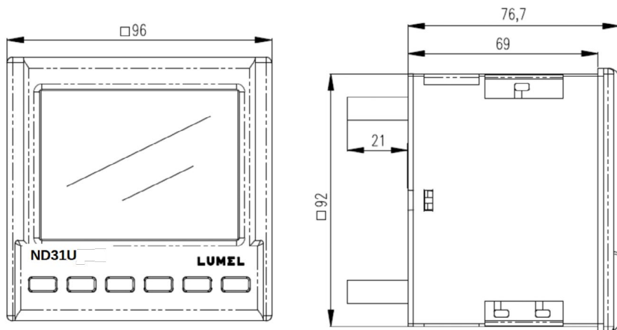
Rys. 3. Rysunek gabarytowy miernika ND31U
